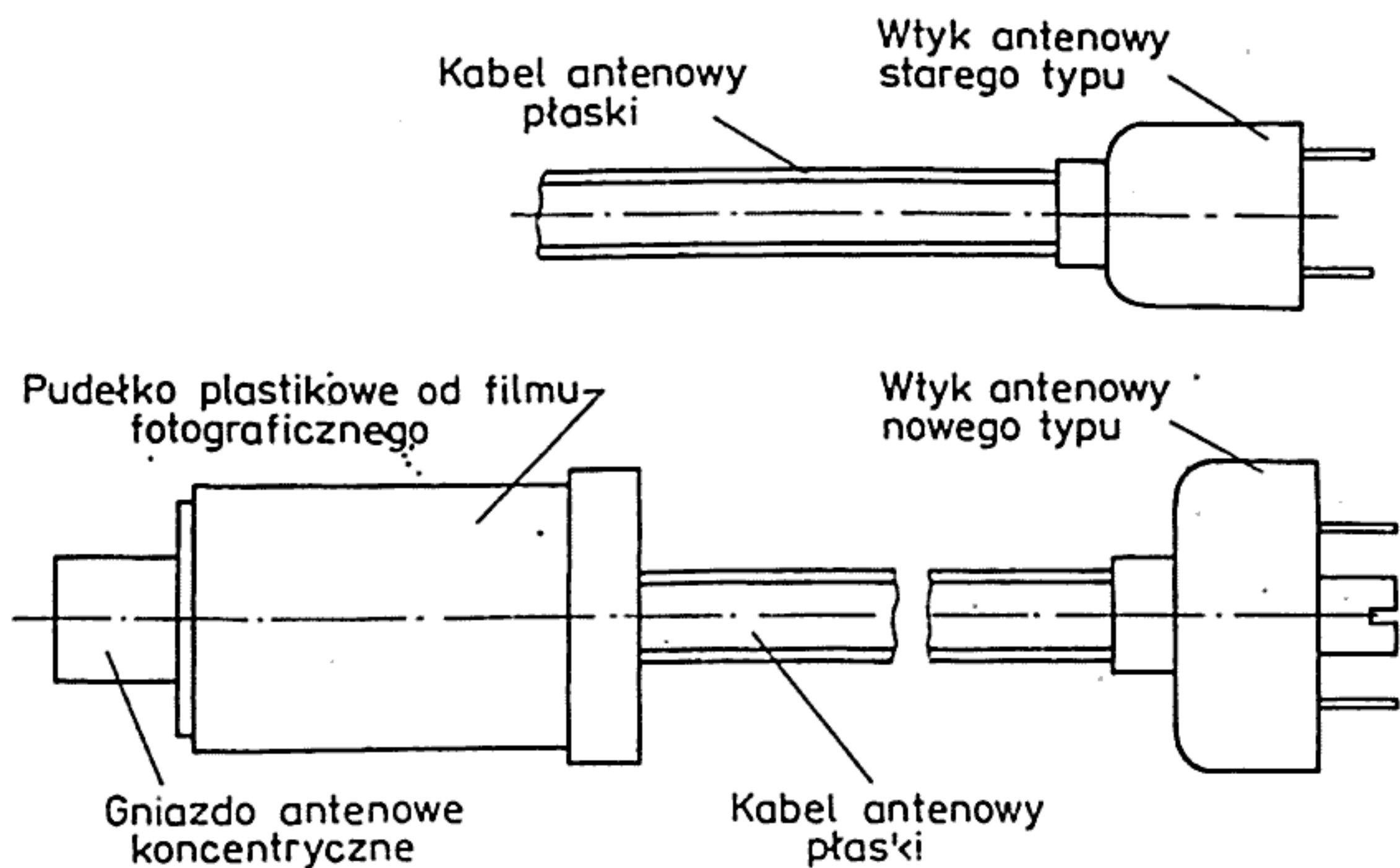
Rys. 1. Złącze przejściowe symetryczne — koncentryczne
