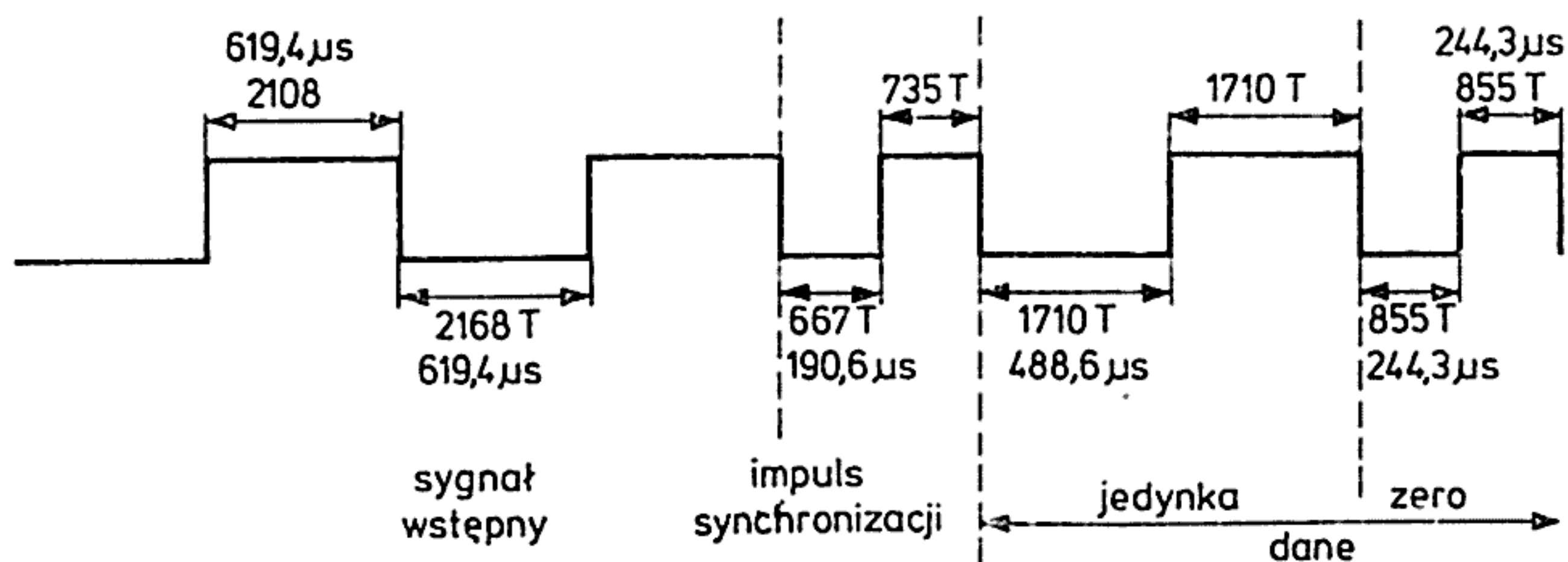
Rys. 25. Sposób zapisu sygnału na taśmie magnetofonowej
