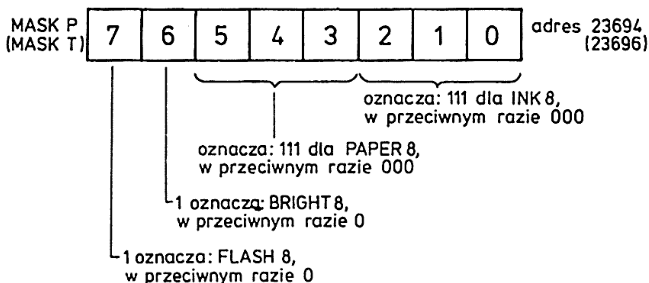
Rys. 12. Organizacja zmiennej systemowej MASK P (MASK T)
