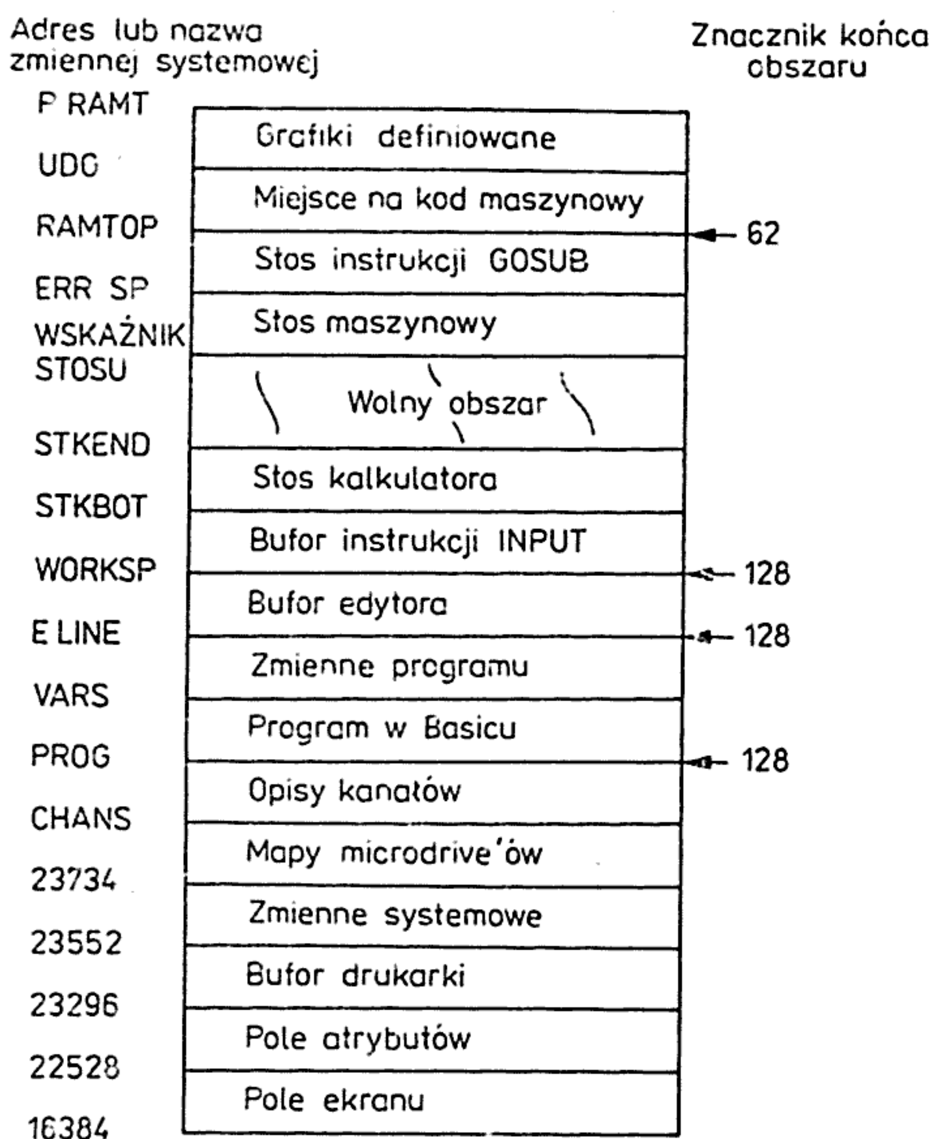
Rys. 24. Mapa pamięci RAM ZX Spectrum
