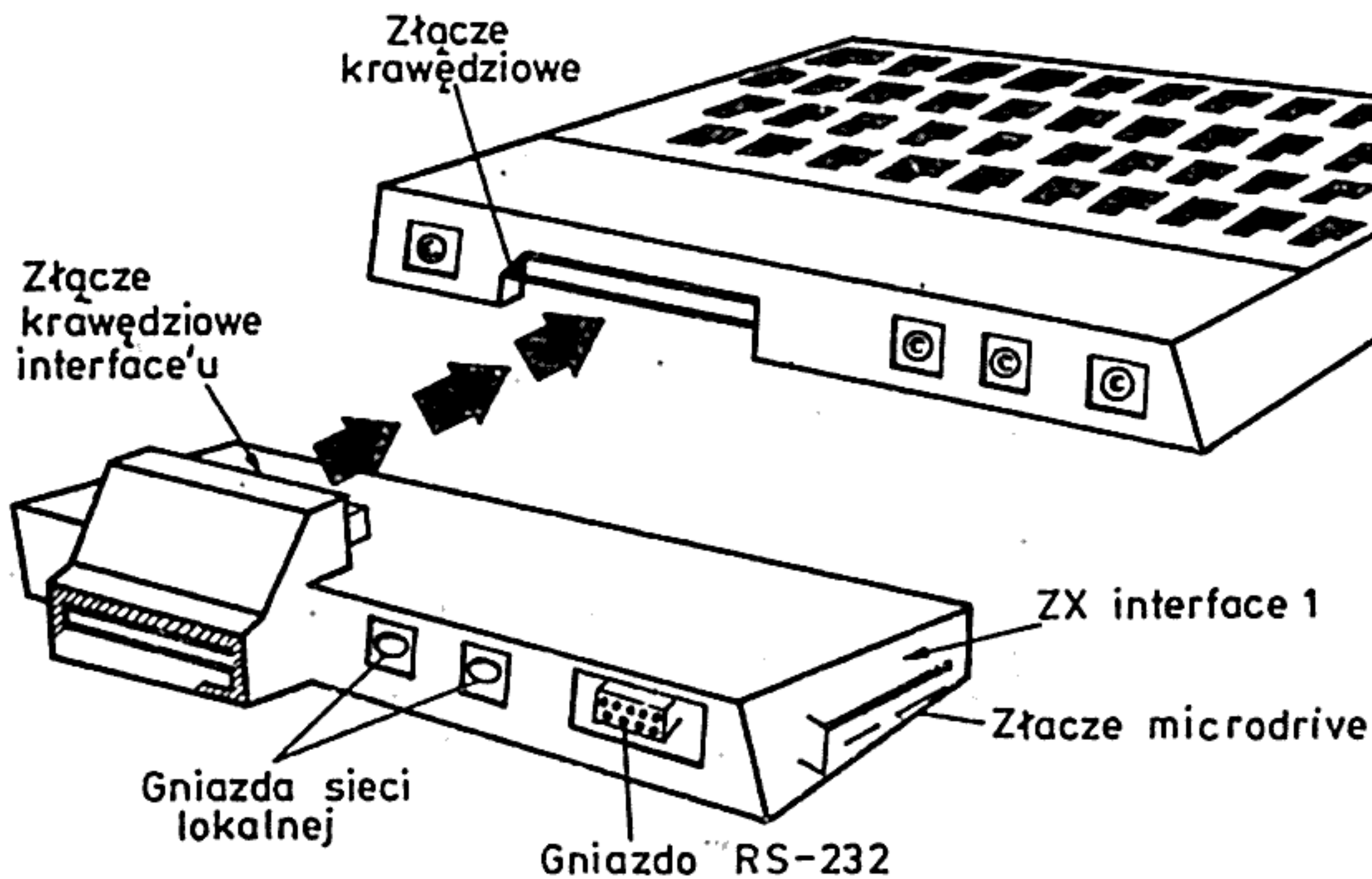
Rys. 28. Sposób połączenia Interface 1 z ZX Spectrum
