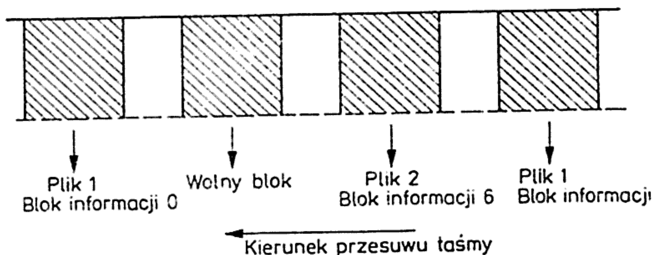
Rys. 32. Organizacja danych na kasetce
