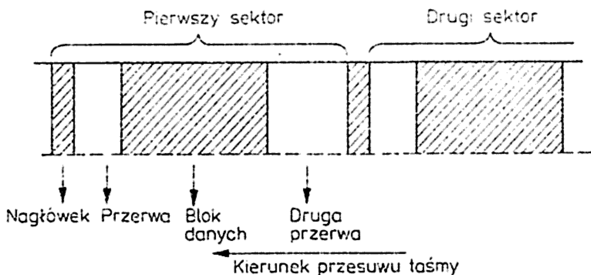
Rys. 31. Sektory zapisane na taśmie microdrive
