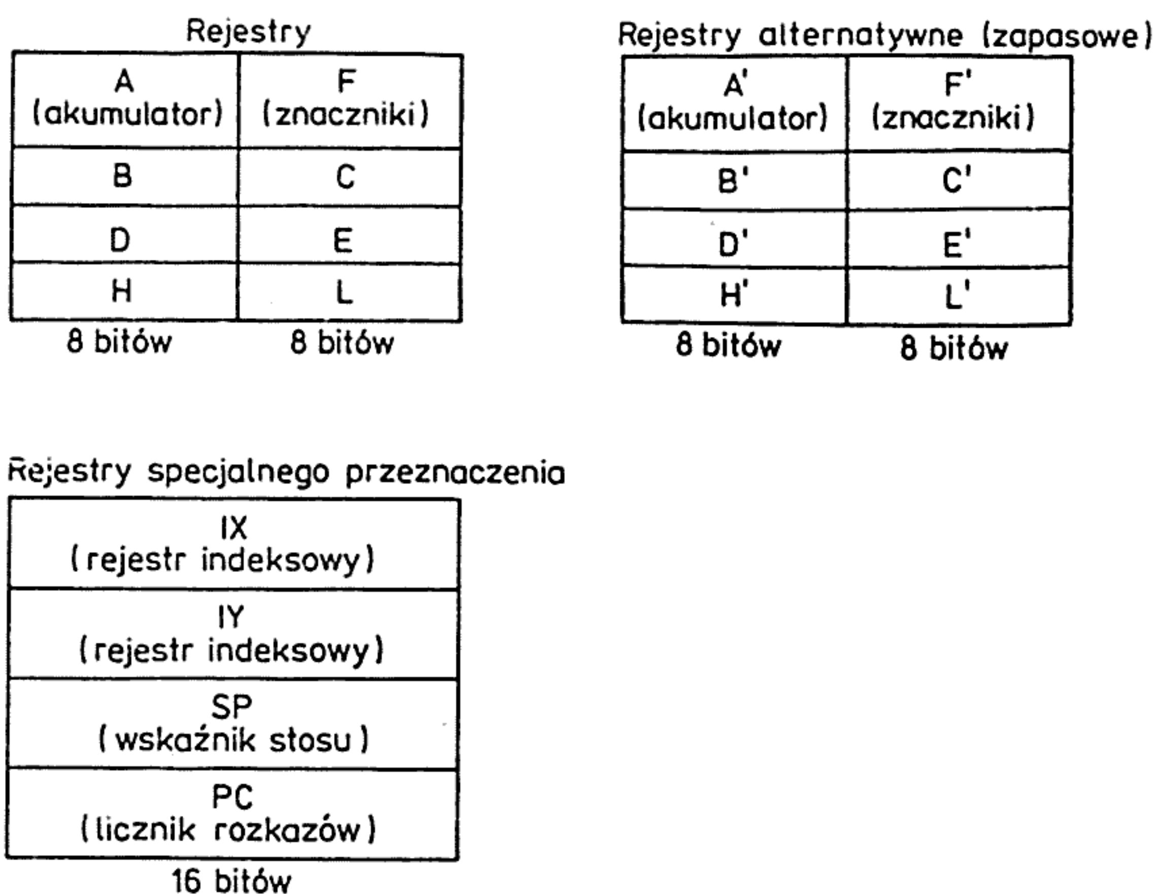
Rys. 23. Rejestry procesora Z80
