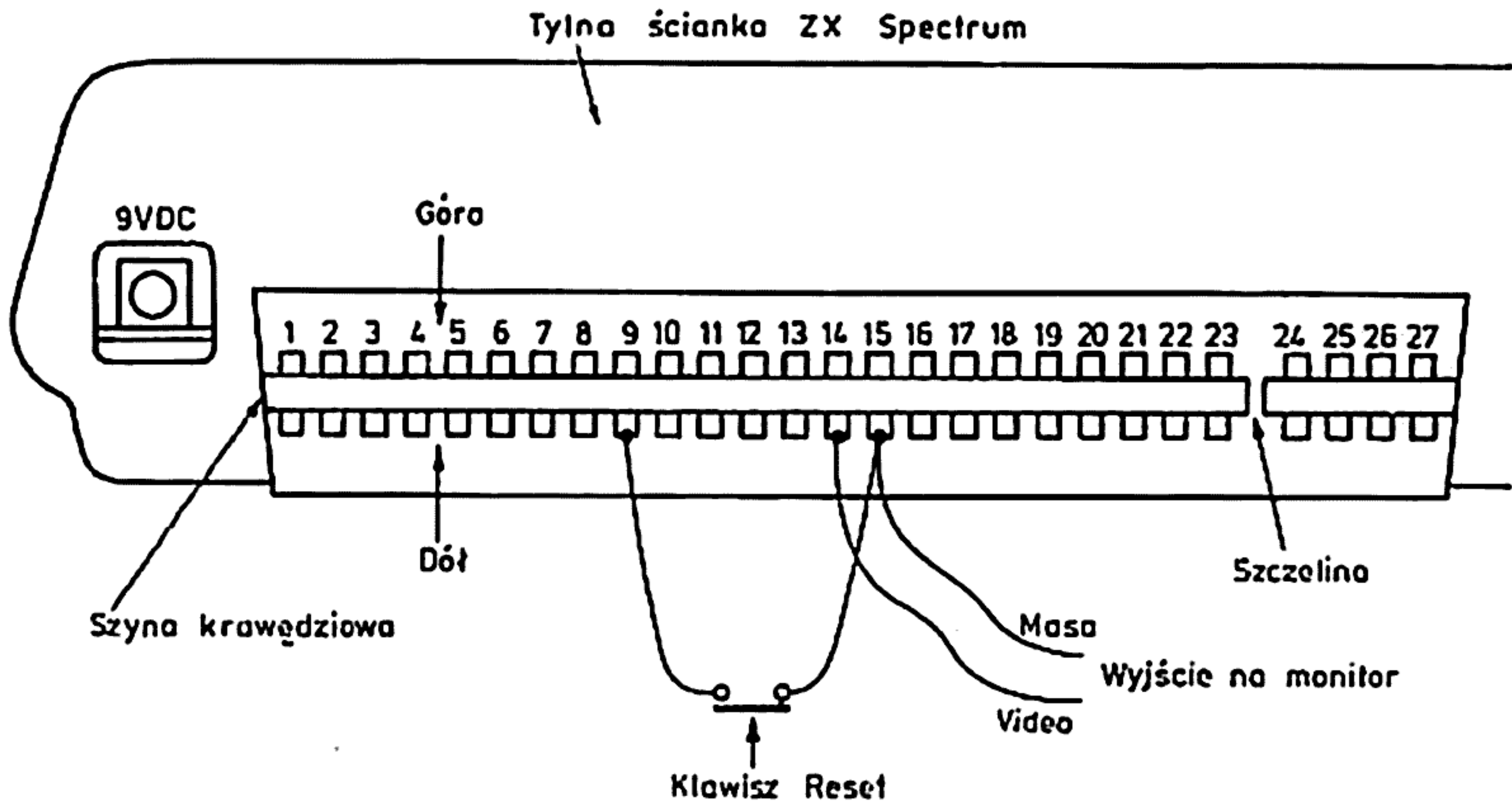
Tablica E. Sygnały na szynie krawędziowej
