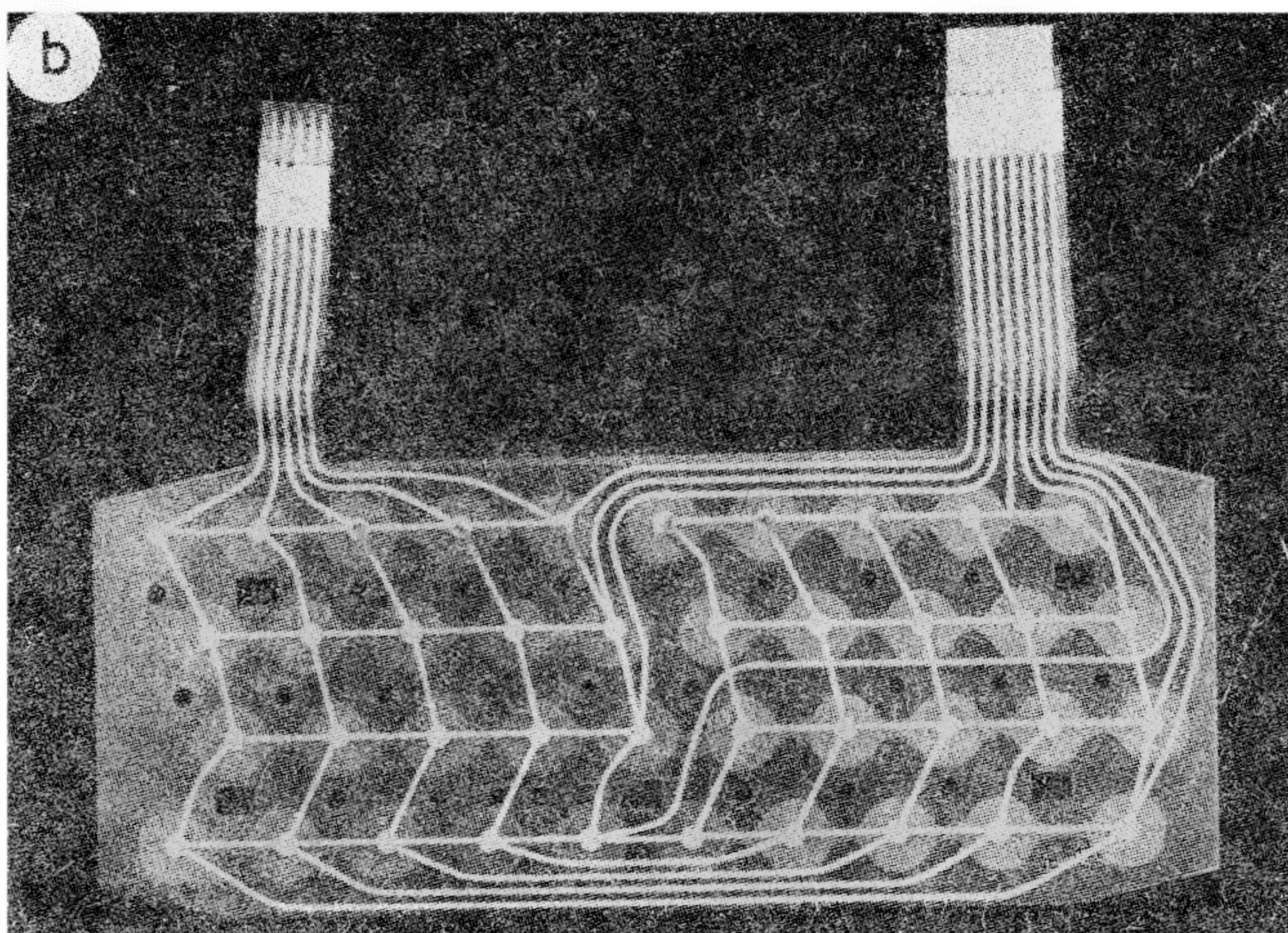
Rys. 8. Klawiatura ZX Spectrum: a — schemat, b — wewnątrz (wygląd)
