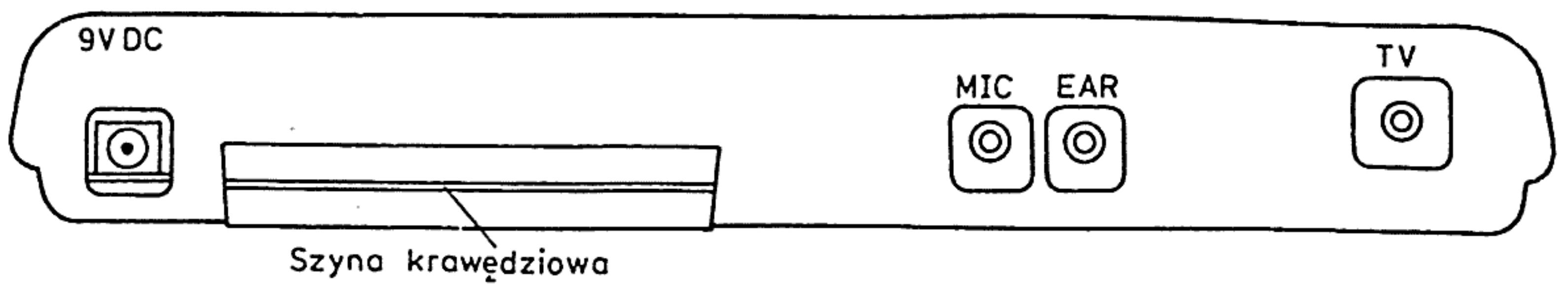
Rys. 6. Tylna ścianka ZX Spectrum
